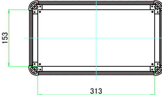
C-C ( 1 : 6 )
