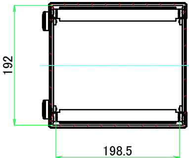
B-B ( 1 : 6 )
